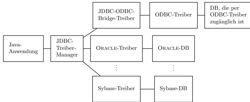
Abbildung 18.1: JDBC-Architektur
